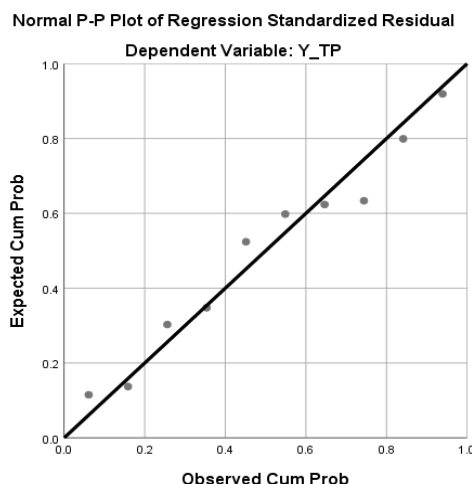
Gambar 1. Uji Normalitas
