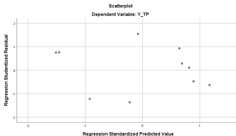
Gambar 2. Uji Heterokedastisitas
